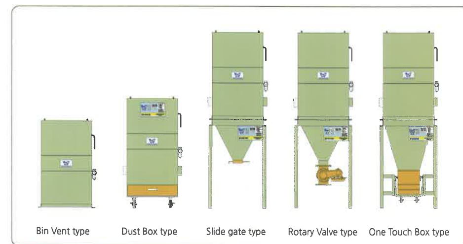
카트리지 집진기 레이아웃
